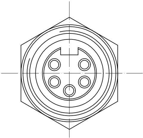
WIDOK OD STRONY CZOLA FRONT SIDE VIEW
